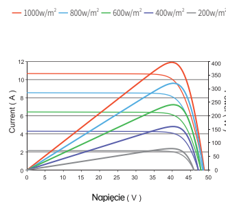
Charakterystyka prądowo - napięciowa (400W)
